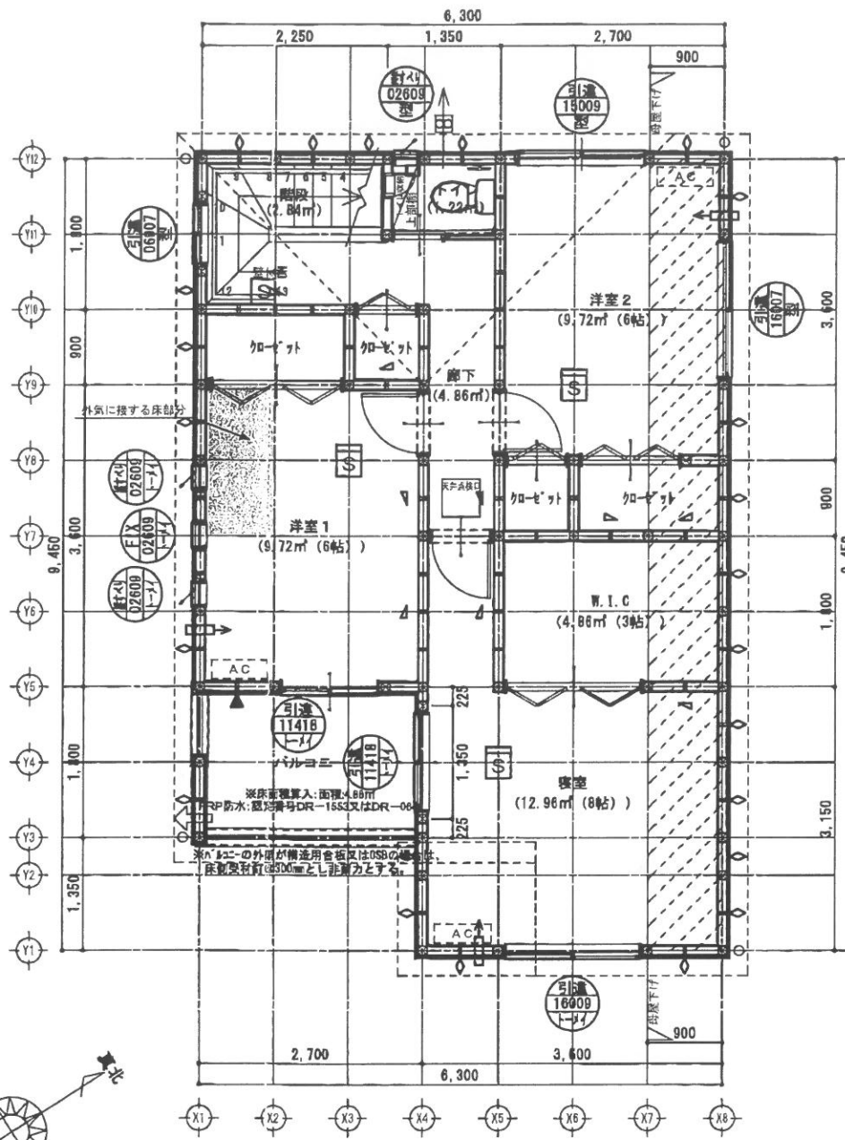
2階平面詳細図 S:1/75
