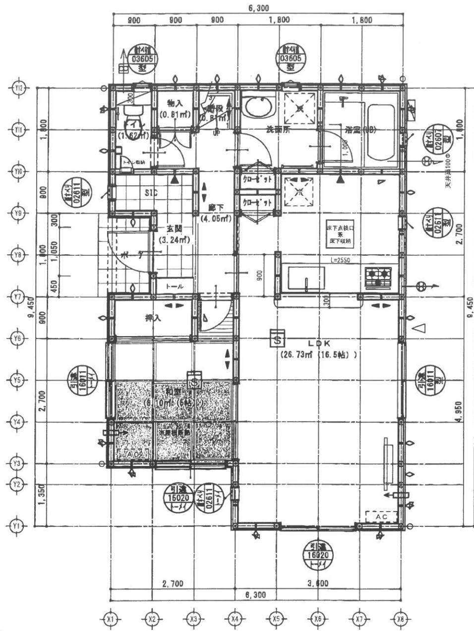
1階平面詳細図 S:1/75
